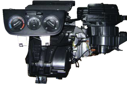
● Air Conditioning System / Klima Sistemi FIAT LINEA (D200)
